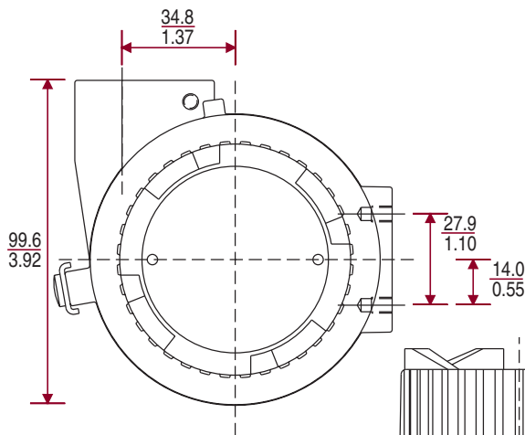
TYPE 2000
